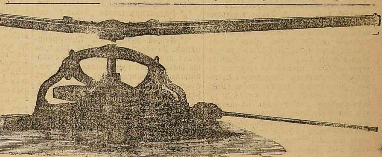
Конный приводъ (типа Клейтона).
