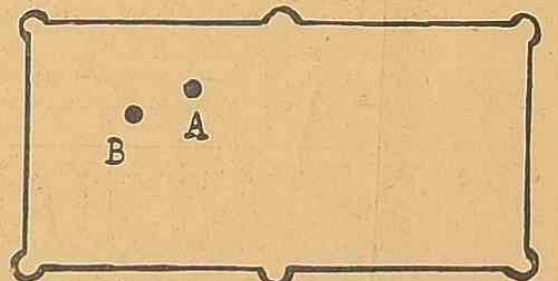
На биллиардномъ полѣ находятся 2 шара А и В. Въ какомъ направленіи необходимо ударить шаръ А, чтобы онъ, ударившись обо всѣ 4 борта биллиарда попалъ въ концъ-концовъ въ шаръ А?
