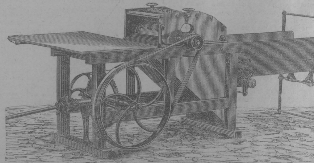
МОЛОТИЛКА ДЕРЕВЯННАЯ СЪ ПЕРЕДАЧЕЙ. Складъ Н. П. Мельникова.
