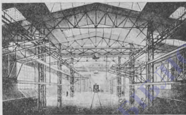
Внутренний вид металлических конструкций цехового здания.
