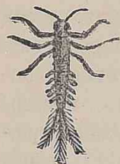
Фиг. 20 Личинка эфемеры (Chloë rufulum).
