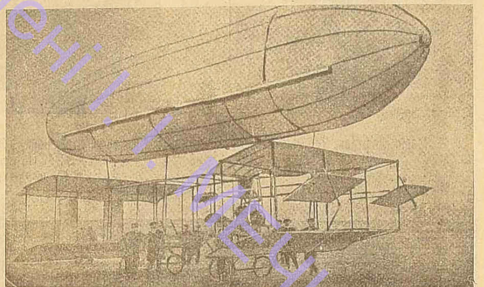
Новая воздухоплавательная машина. — Комбинація дирижабля съ двумя бипланами. Изобрѣтеніе французскаго инженера Сезари.
