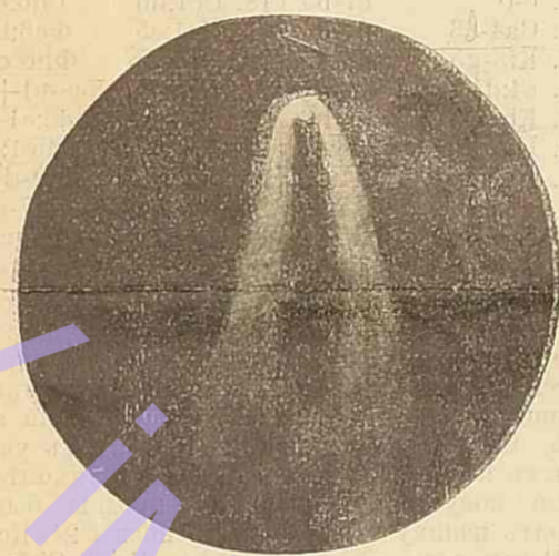
Новая комета („1910 А“). Съ фотографическаго снимка кембриджской обсерваторіи.
